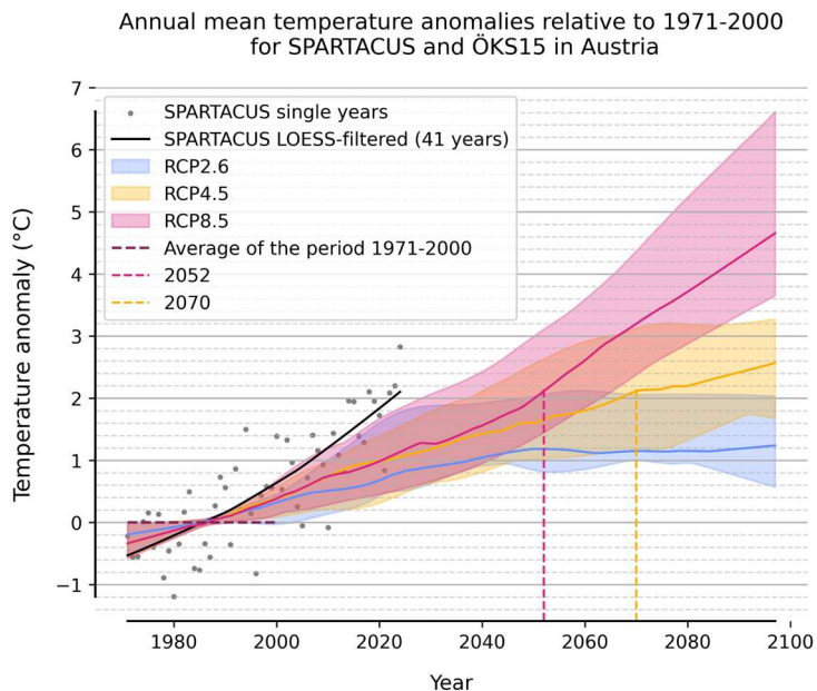
Abb 3: Beobachteter Temperaturtrend (schwarz) und modellierte Trends (farbig schattiert, Median der Modelle als farbige Linien) in Österreich, relativ zur Periode 1971-2000. Die vertikalen, gestrichelten Linien geben die gewichtete Mitte des Zeitraums an, in dem das Temperaturniveau von 2024 erreicht wird (Abb. übernommen von Box 1.1 Figure 2 in AAR2, Kapitel 1 ).
