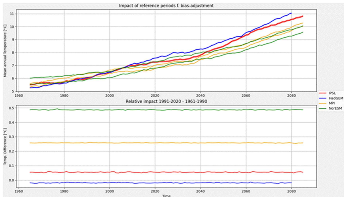
Abb 1: Unterschiede Bias-Korrektur (mit Scaled Distribution Mapping) 1961-1990 vs. 1991-2020. Simulationen: EURO-CORDEX, 1 Modell angetrieben von 4 verschiedenen GCMs.
